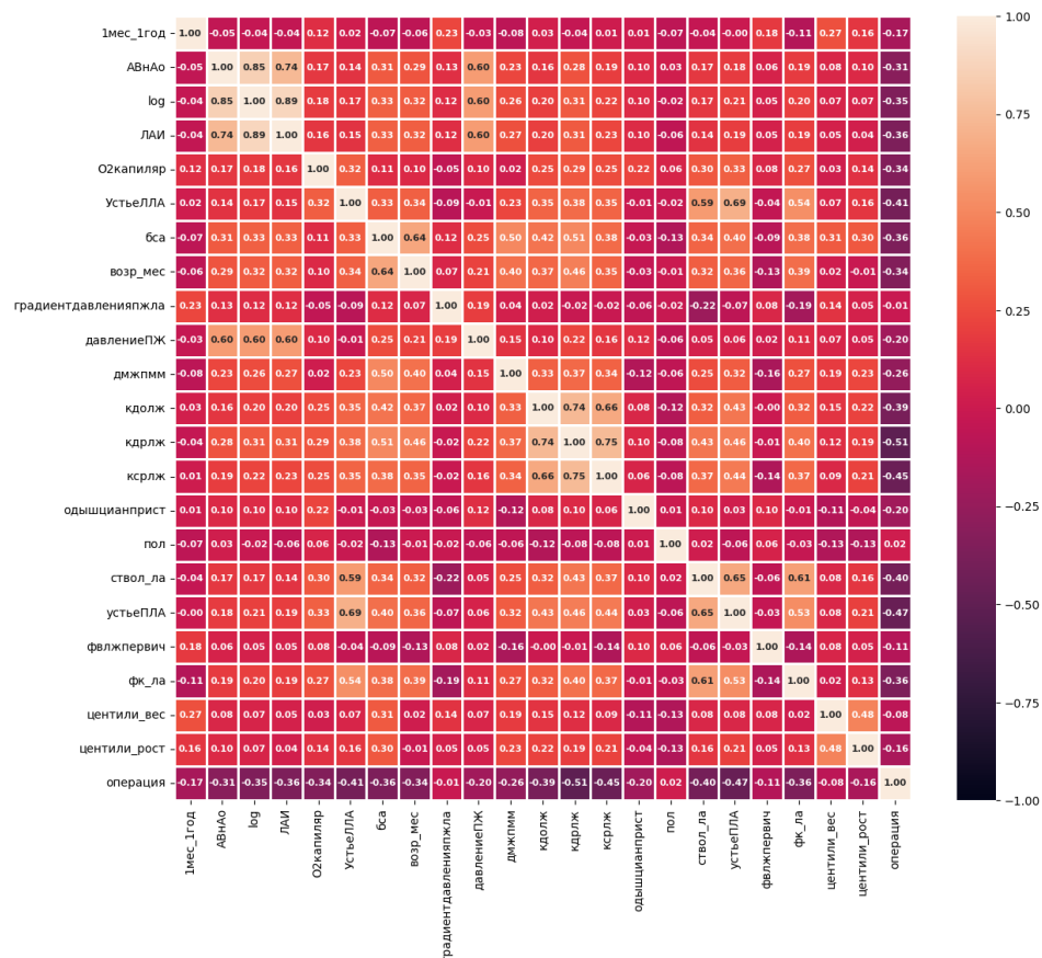
Рисунок 4. Попарный анализ мультиколлинеарности с помощью коэффициента ранговой корреляции Кендалла
