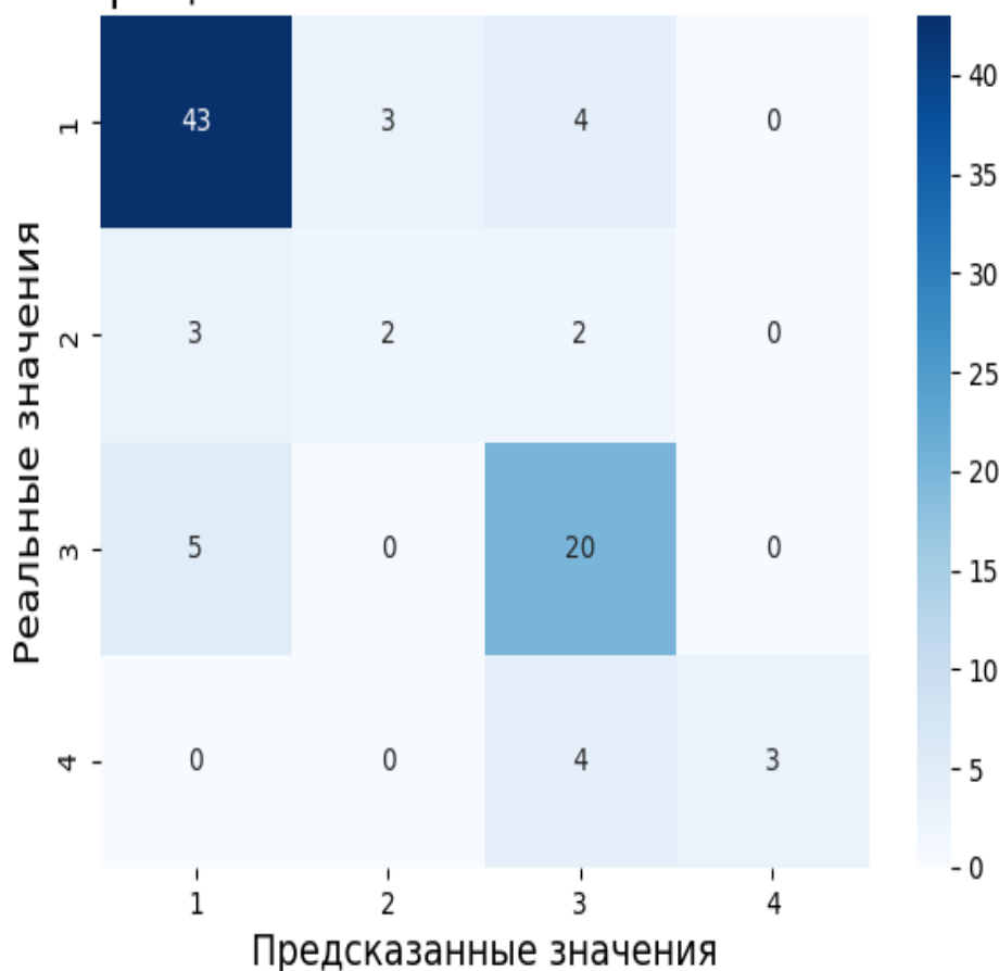
Матрица ошибок RandomForestClassifier
