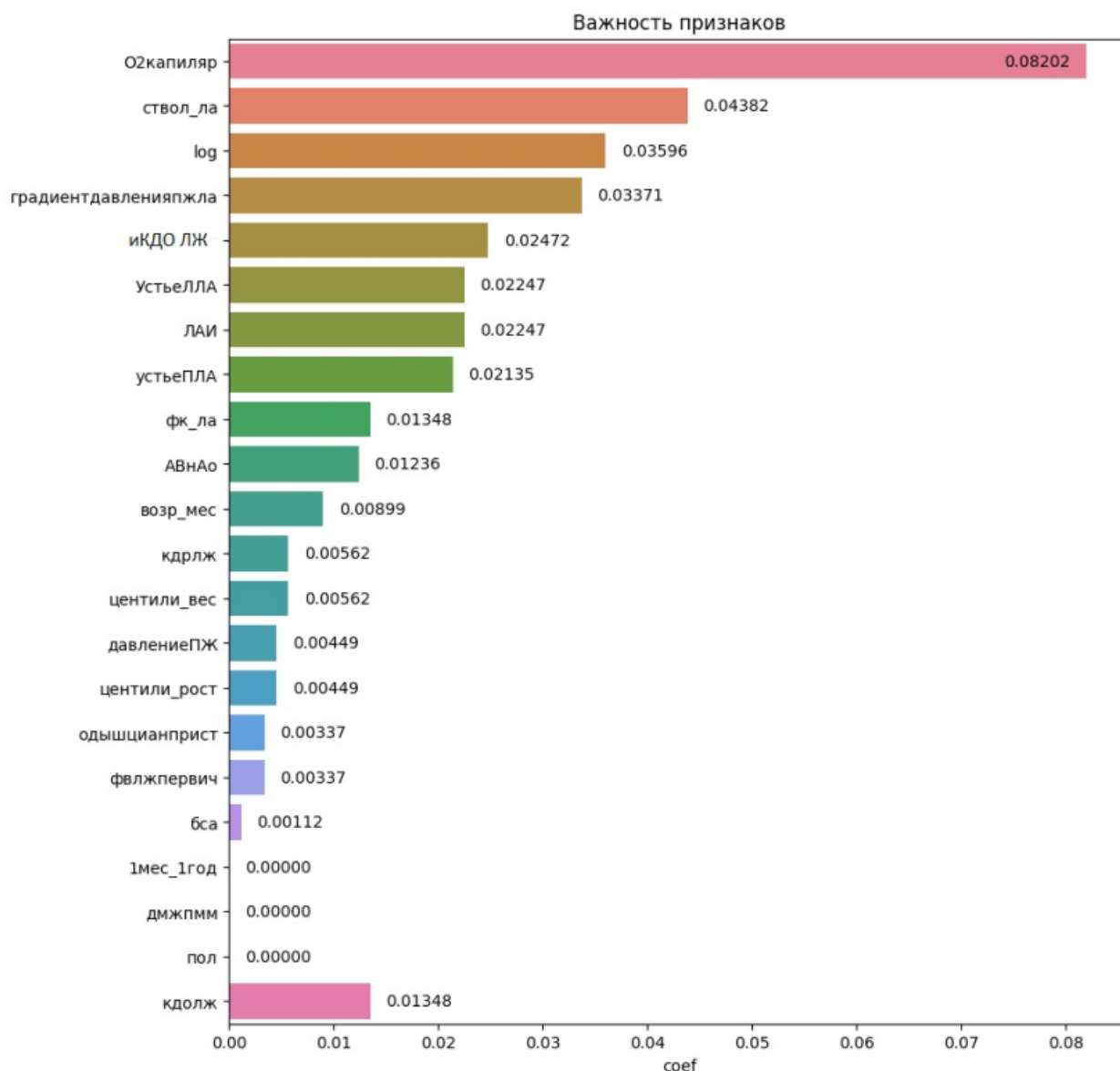
Рисунок 12. Важность признаков для моделей машинного обучения.
