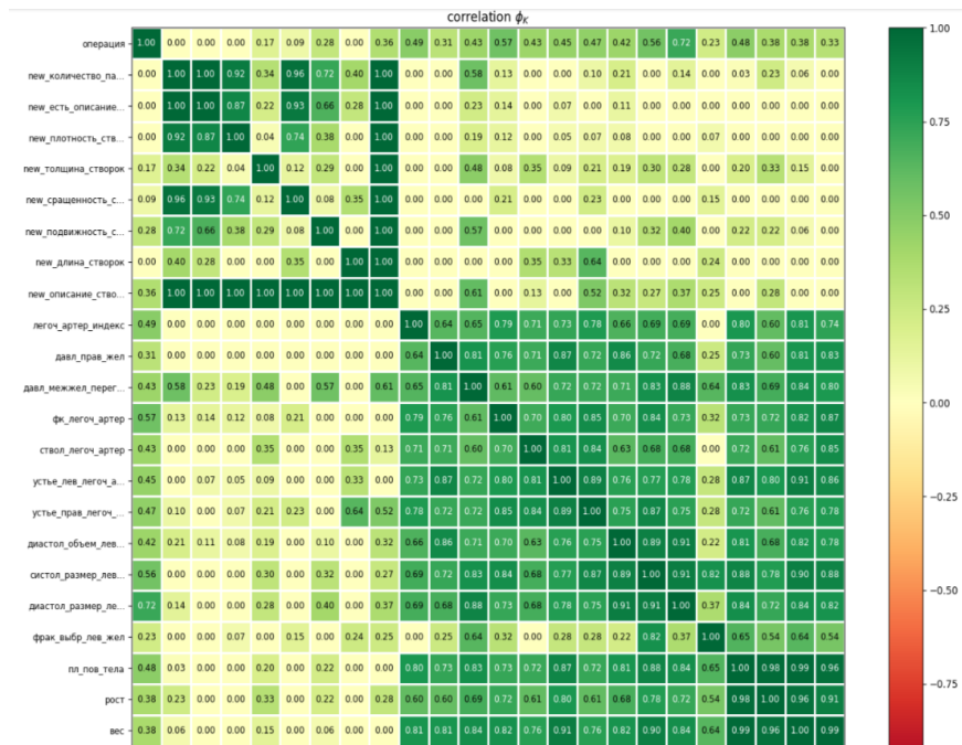
Рисунок 3. Проверка признаков на мультиколлинеарность с целевым признаком.
