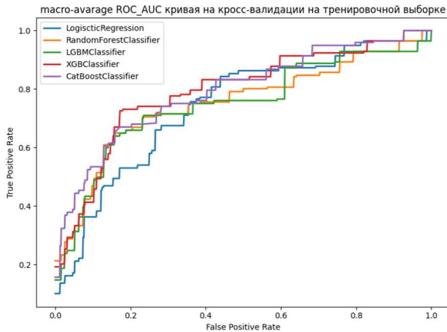
Рисунок 6. ROC- кривые сравнения всех используемых моделей МО.
