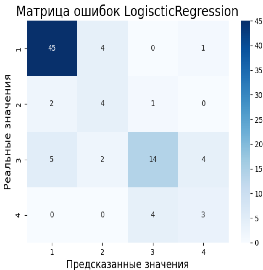
Рисунок 9. Матрица ошибок модели машинного обучения Logistic Regression
