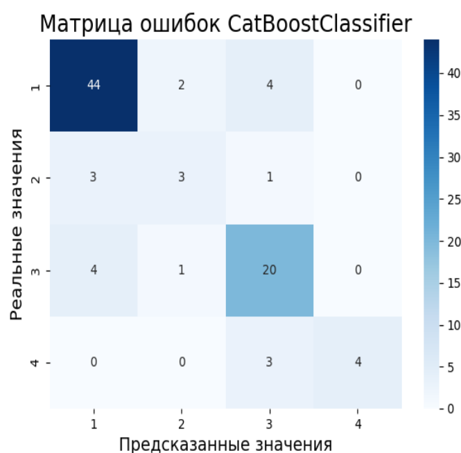
Рисунок 8. Матрица ошибок модели машинного обучения CatBoostClassifier.
