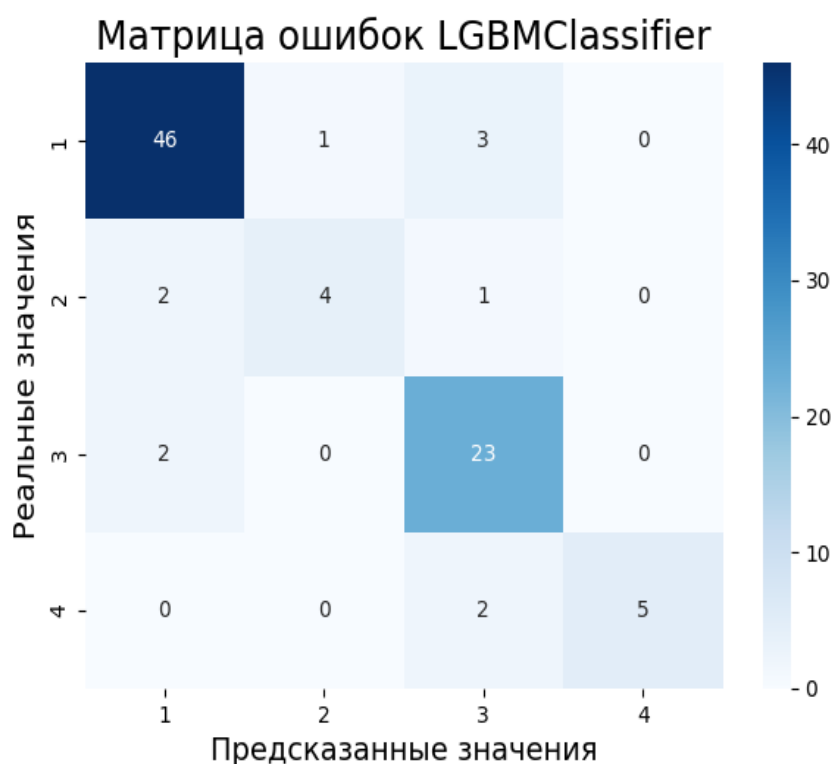
Рисунок 7. Матрица ошибок модели машинного обучения LGBM Classifier
